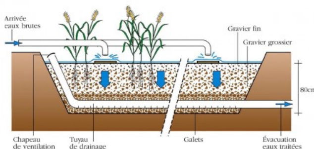
Station de traitement type filtre planté de roseaux
